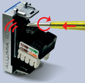
Sgancio Uncoupling
