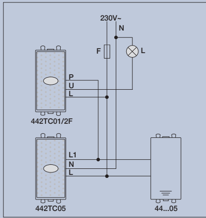
L: carico L: load F: fusibile tipo F 2A H 250V~ F: fuse type F 2A H 250V~
