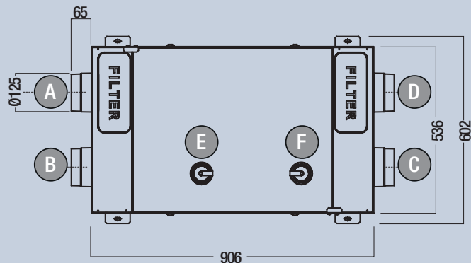
Vista dall'alto View from above
